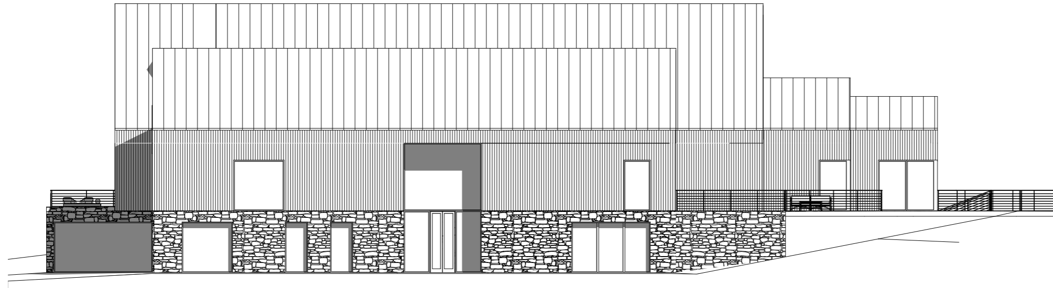
FASAD MOT VÄSTER
